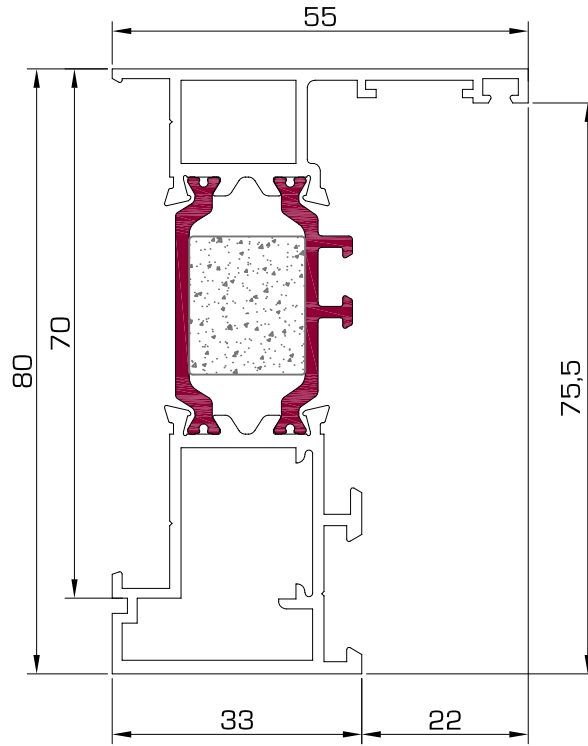
6006 Marco guía renovación
