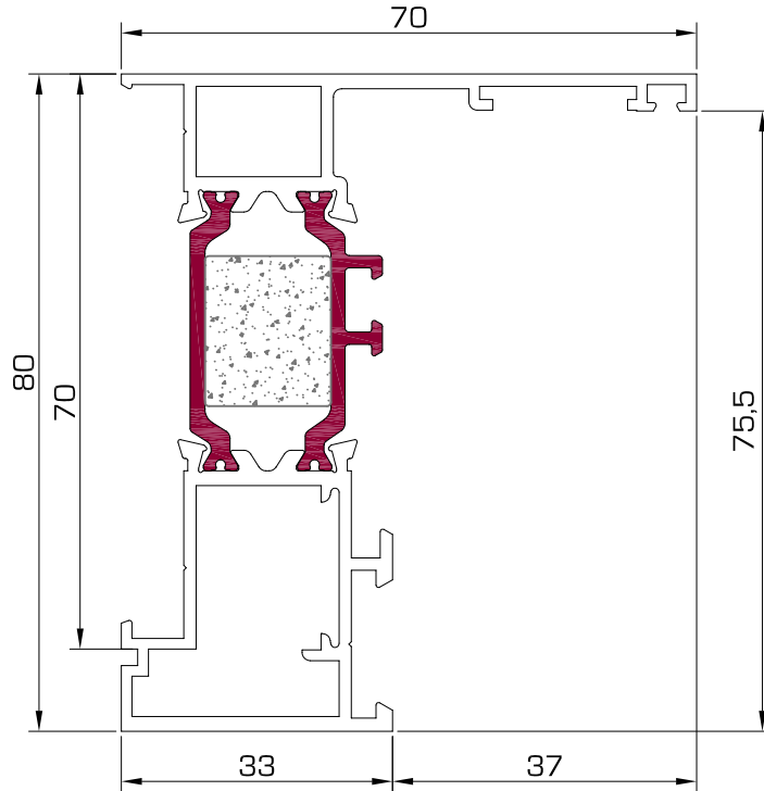
6056 Marco guía renovación H.O.
