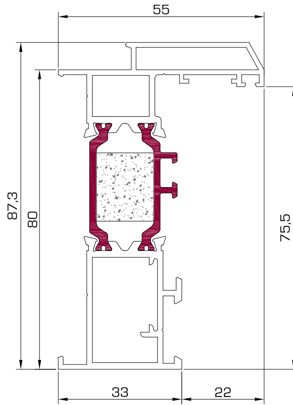
6007 Marco desagüe oculto
