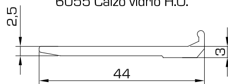
6055 Calzo vidrio H.O.
